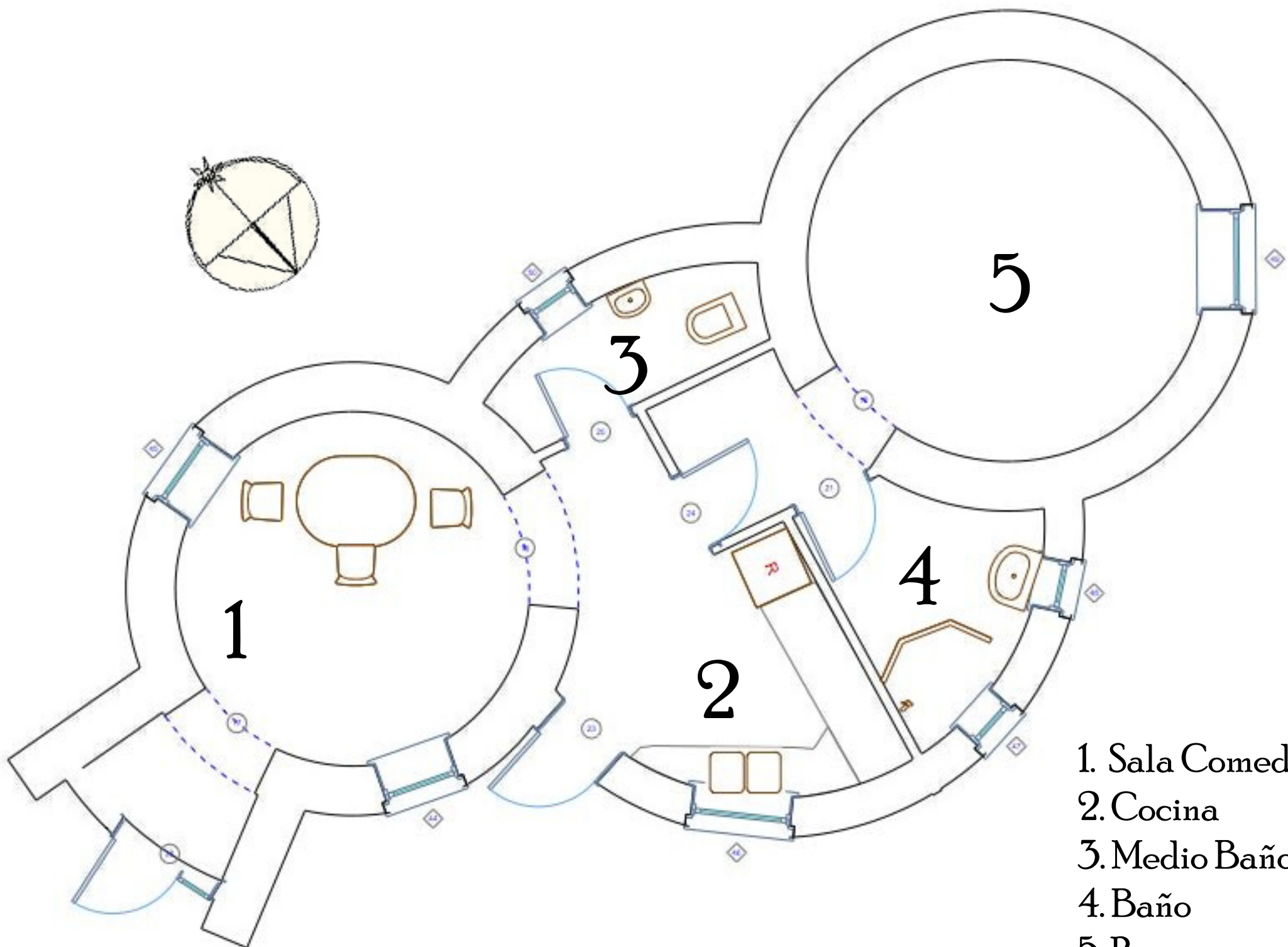
PLANTA ARQUITECTÓNICA
