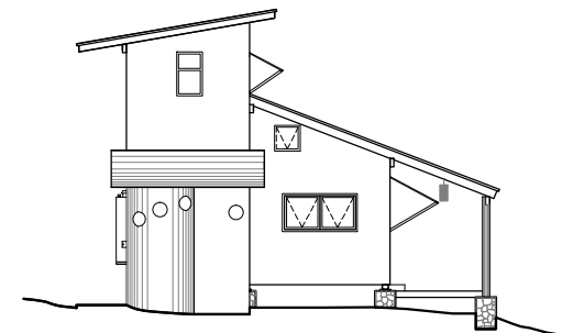
FACHADA LONGITUDINAL
