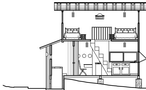
CORTE X-X'
