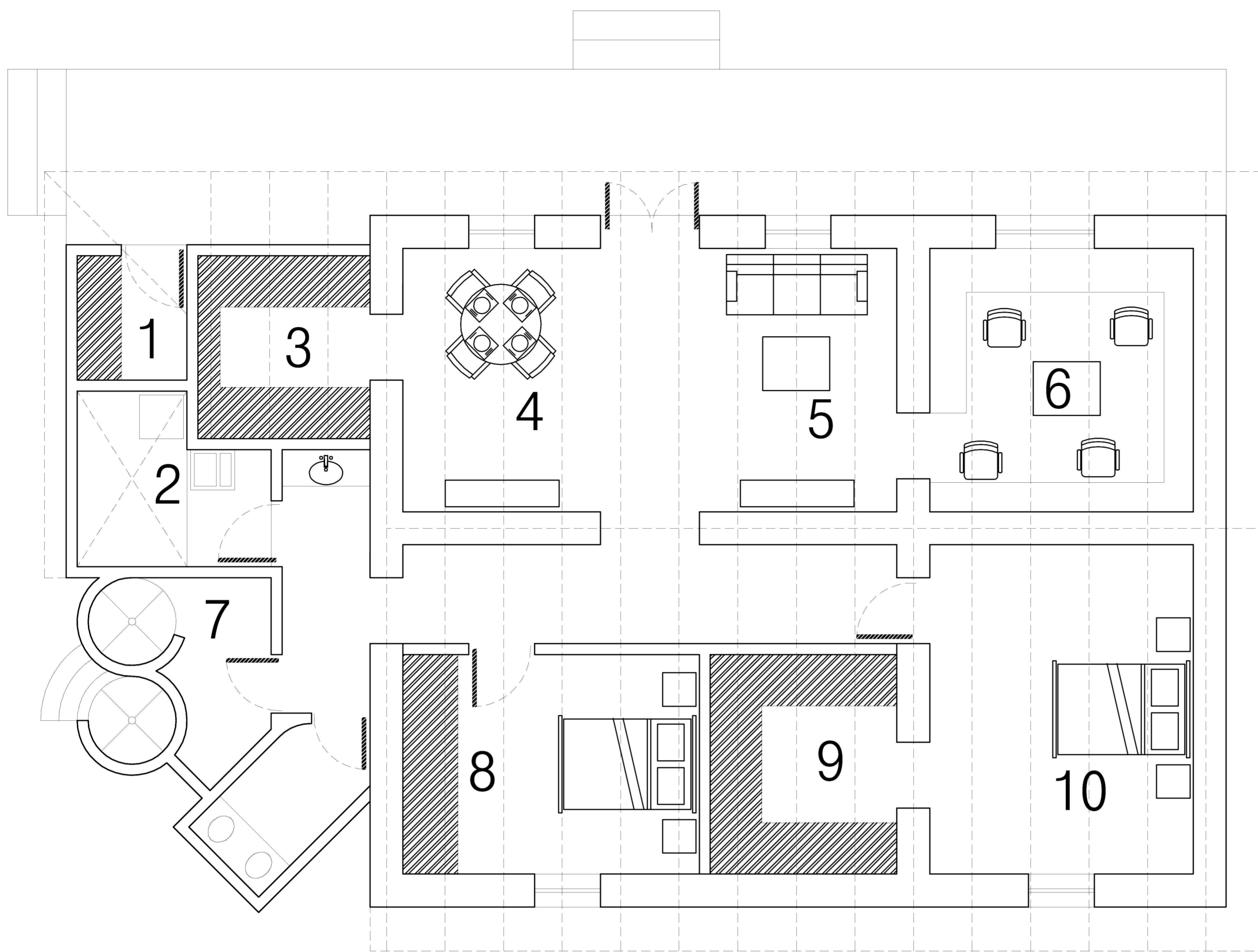
PLANTA ARQUITECTÓNICA
