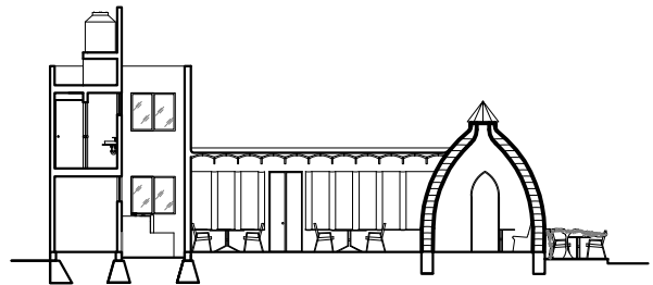
CORTE LONGITUDINAL X-X'
